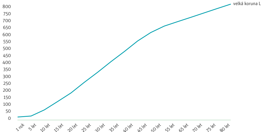
Graf 4 Růstová křivka pro stromy s velkou korunou (L) v prostředí městské ulice, objem koruny stromů v m³ uveden na ose y
