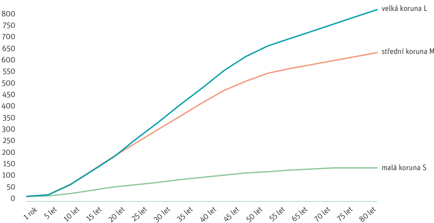
Graf 1 Vzájemné srovnání růstových křivek jednotlivých kategorií stromů, objem koruny stromů v m³ uveden na ose y
